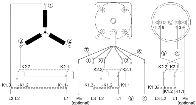
Bild 3: Dreiphasen-Motor, Schaltungsvorschlag zum Ein-/Ausschalten und Reversieren mit mechanischen Kontakten
